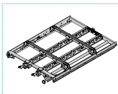
302. BOVENSEPARATIERAAM MET QUICK-LOCK
