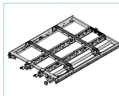
302. BOVENSEPARATIERAAM MET QUICK-LOCK
