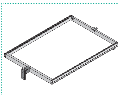
321. ONDERSTE SCHUIFRAAM
