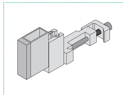
332. UITDUWER Lengte = 50 mm
