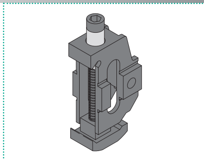
270. KLEMSTUK
