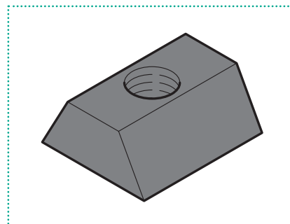
351. ZWALUWSTAARTMOER M 8 (groot model)
