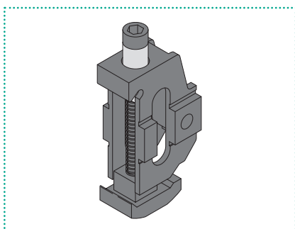
270. KLEMSTUK
